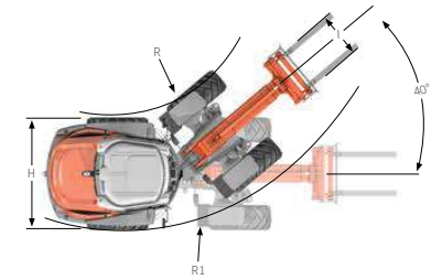
Mit Palettengabel
